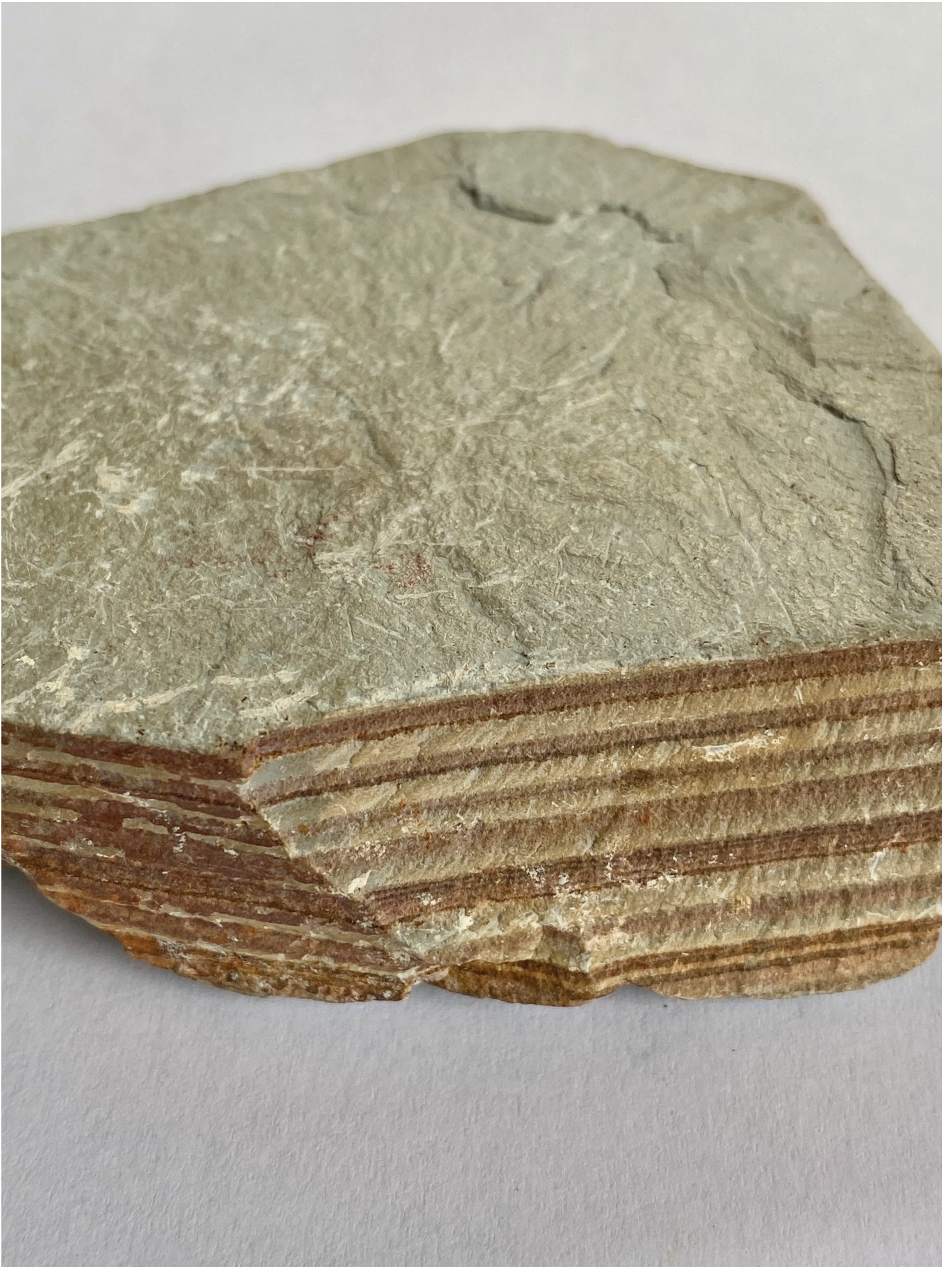
Pelitas / Ritmitas
