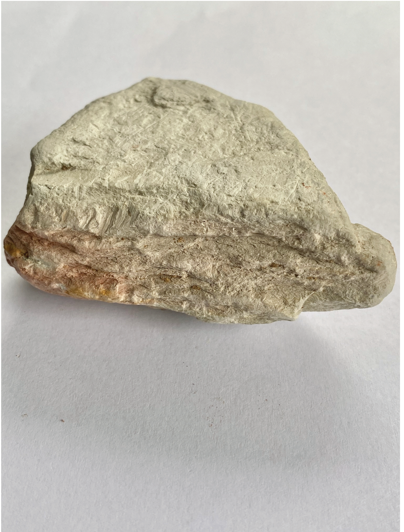
Limolitas
